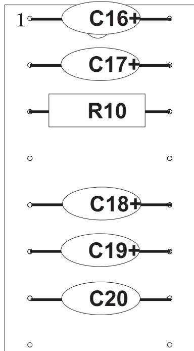
Soquete 16pinos
