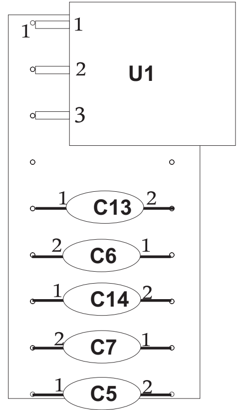
Soquete 18pinos
