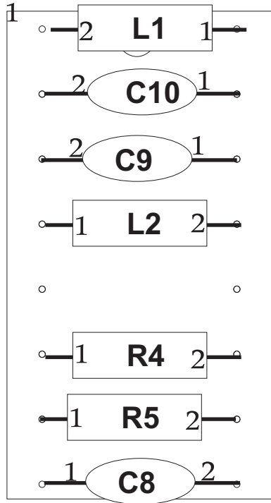
Soquete 16pinos
